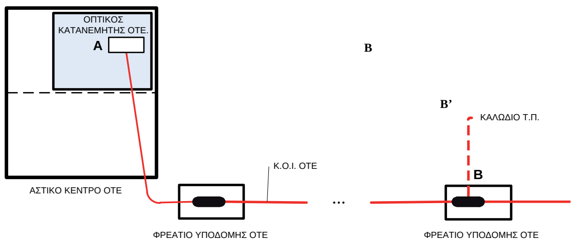
Σχήμα 2. Διάγραμμα παροχής Οπτικής ίνας ΟΤΕ σε Τ.Π.. Ο Τ.Π. παραλαμβάνει την Οπτική Ίνα στα σημεία Α και Β.
