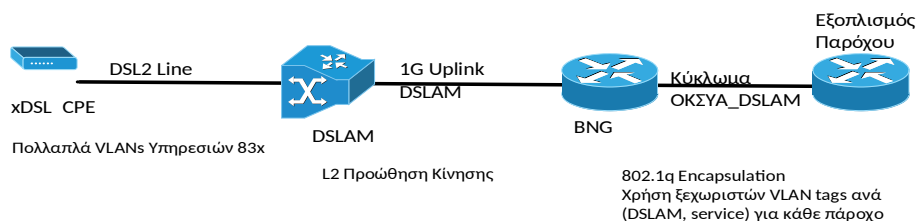
Σχήμα 1: Τοπολογία VPU / VPU light
