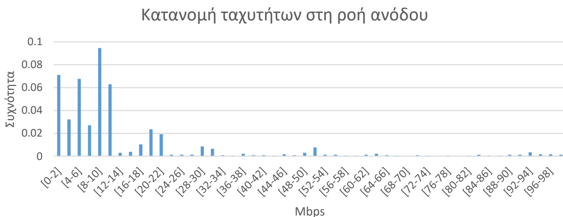
Σχήμα 2 Κατανομή ταχυτήτων στη ροή καθόδου και στη ροή ανόδου, για τις μετρήσεις στον ΥΠΕΡΙΩΝ το 2024
