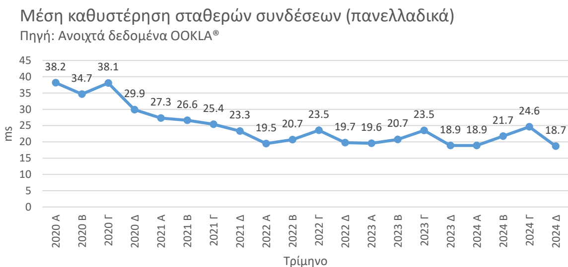
Σχήμα 9 Μέση ταχύτητα σταθερών συνδέσεων σε πανελλαδικό επίπεδο ανά τρίμηνο τα έτη 2020-2024.
