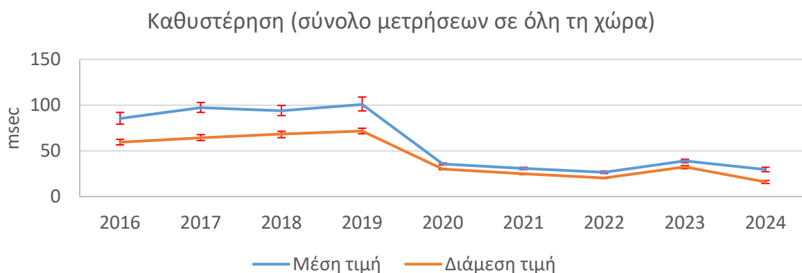
Σχήμα 6. Εξέλιξη της μέσης και μεσαίας τιμής της καθυστέρησης (RTT) από το 2016 έως και το 2024 σε πανελλαδικό επίπεδο.
