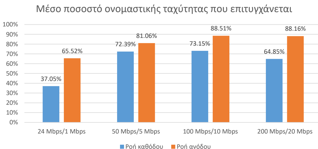
Σχήμα 4 Μέσο ποσοστό ονομαστικής ταχύτητας που επιτυγχάνεται για τα δημοφιλέστερα πακέτα με βάση τις μετρήσεις του ΥΠΕΡΙΩΝ για το 2024.
