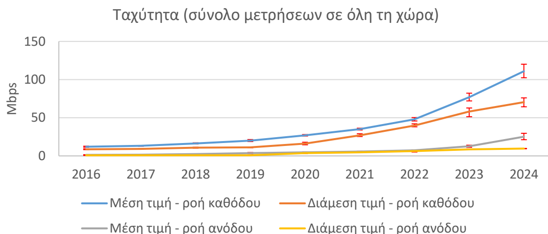
Σχήμα 5. Εξέλιξη της μέσης και μεσαίας τιμής των ταχυτήτων στη ροή καθόδου και ανόδου από το 2016 έως και το 2024 σε πανελλαδικό επίπεδο.
