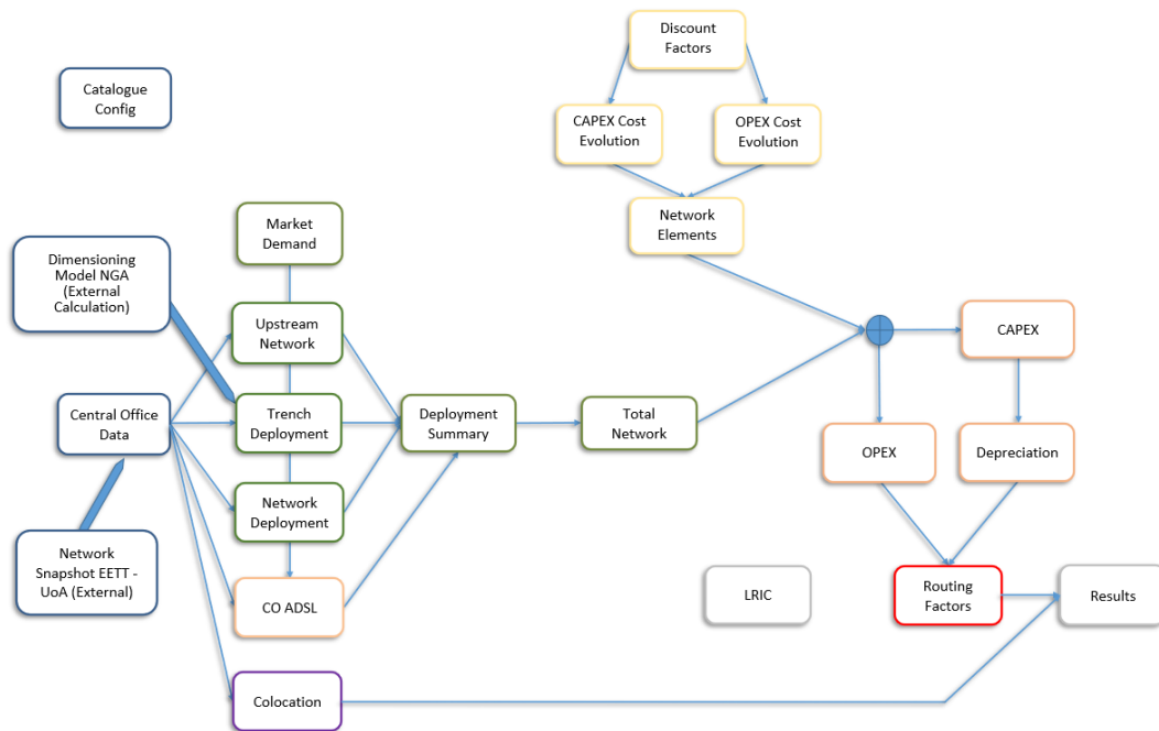
Σχήμα 3-1: Δομή αρχείου bottom_up_model
