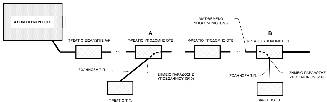
Σχήμα 2. Διάγραμμα παροχής σωληνώσεων ΟΤΕ σε Τ.Π.. Ο Τ.Π. παραλαμβάνει σωλήνωση από τα σημεία Α & Β (Φρεάτια υποδομής ΟΤΕ που βρίσκονται πλησιέστερα στα σημεία επιλογής του Τ.Π.). Τα φρεάτια αλλά και η παρεχόμενη σωλήνωση βρίσκονται εντός διαδρομής από το Α/Κ ΟΤΕ έως την Καμπίνα FTTC/FTTH όπως αυτή απεικονίζεται στη βάση ΧΕΜΔ.
