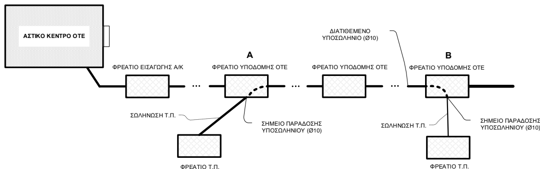
Σχήμα 1. Διάγραμμα παροχής σωληνώσεων ΟΤΕ σε Τ.Π. Ο Τ.Π. παραλαμβάνει σωλήνωση από τα σημεία A & B (Φρεάτια υποδομής ΟΤΕ που βρίσκονται πλησιέστερα στα σημεία επιλογής του Τ.Π.). Τα φρεάτια αλλά και η παρεχόμενη σωλήνωση βρίσκονται εντός διαδρομής όπως αυτή απεικονίζεται στη βάση ΧΕΜΔ.
