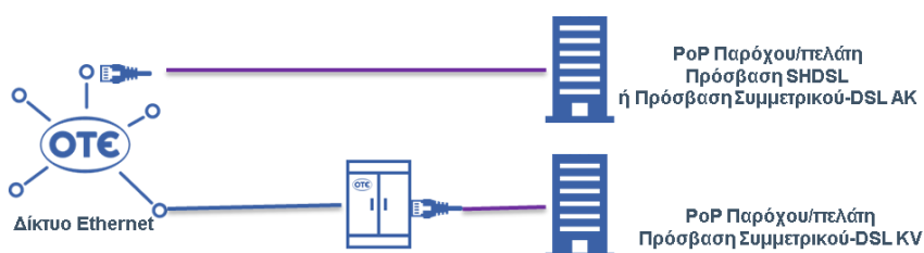
Εικόνα 2: Σχηματική απεικόνιση προσβάσεων Ethernet Χαλκού
