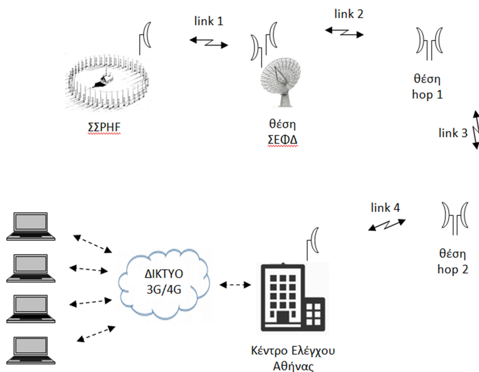
Σχήμα 2: Γενική αρχιτεκτονική δικτύωσης και τρόπου ελέγχου του ΣΣΡΗΦ από το κέντρο ελέγχου της Αναθέτουσας Αρχής στην Αθήνα και τέσσερις (4) φορητούς υπολογιστές.
