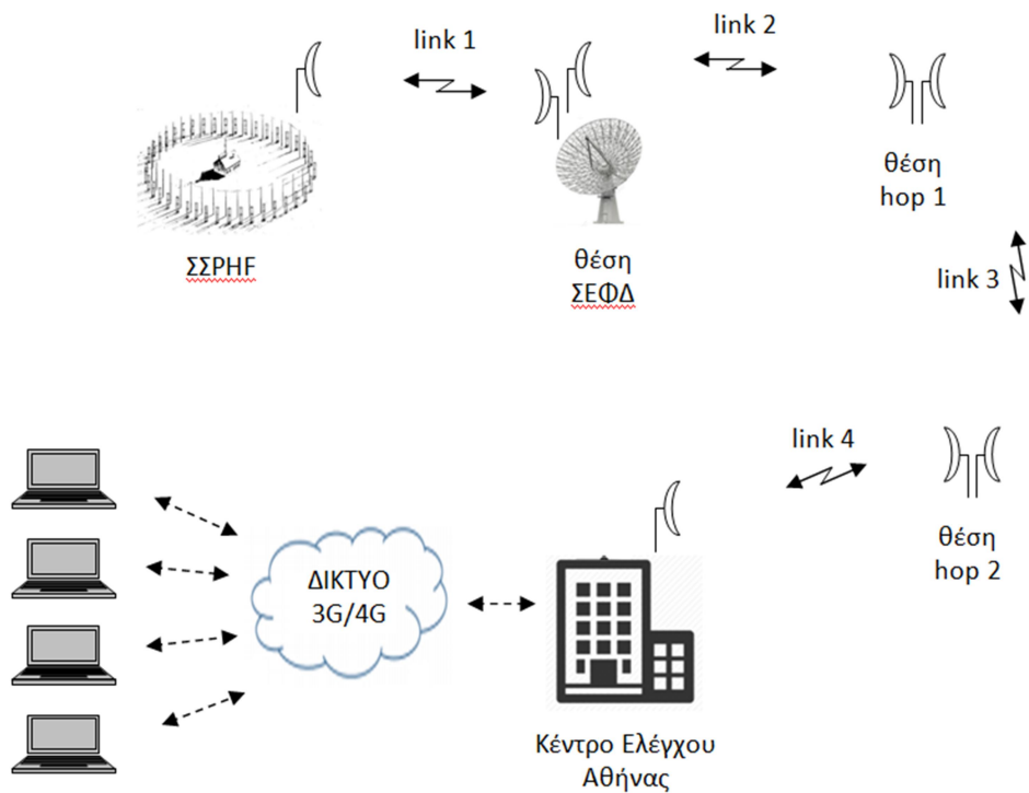
Σχήμα 1: Γενική αρχιτεκτονική δικτύωσης και τρόπου ελέγχου του ΣΣΡΗΦ από το κέντρο ελέγχου της Αναθέτουσας Αρχής στην Αθήνα και τέσσερις (4) φορητούς υπολογιστές.
