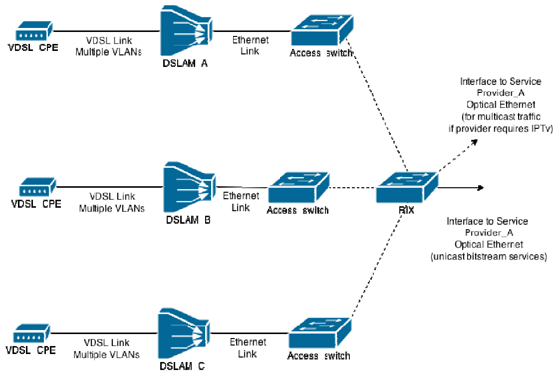
Σχήμα 1 Τοπολογία Bitstream
