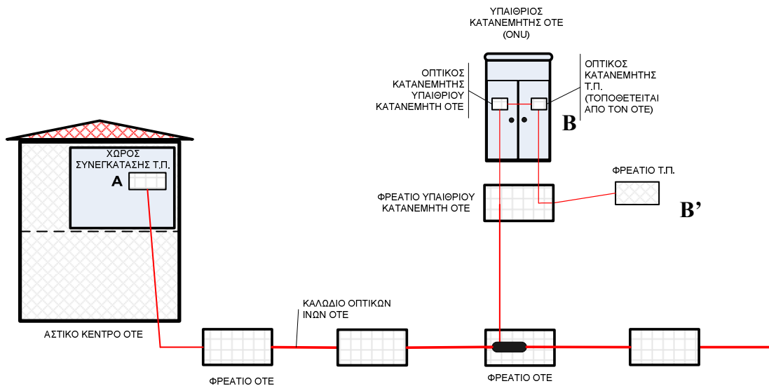
Σχήμα 2. Διάγραμμα παροχής Οπτικής ίνας ΟΤΕ σε Τ.Π.. Ο Τ.Π. παραλαμβάνει την Οπτική Ίνα στα σημεία A και B.
