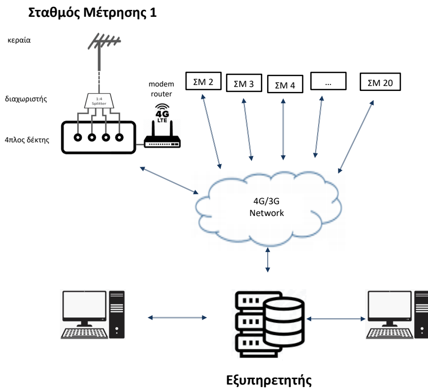
Σχήμα 1: Γενική αρχιτεκτονική συστήματος μέτρησης ποιότητας υπηρεσίας ψηφιακής τηλεοπτικής ευρυεκπομπής
