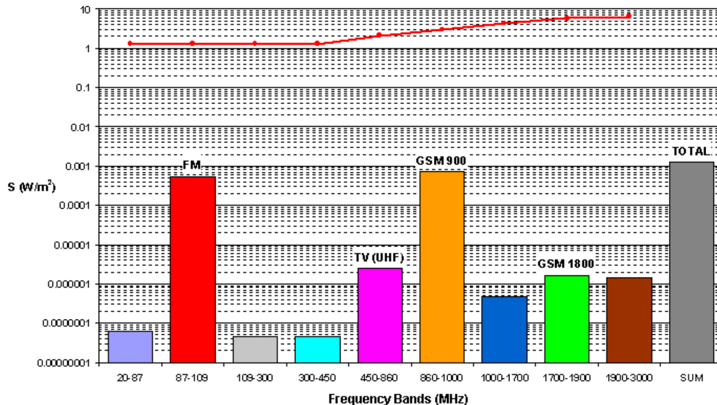
Παρουσίαση πυκνότητας ισχύος κατά συχνοτική περιοχή (ή εφαρμογή)
