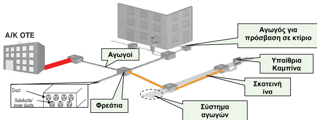
Σχήμα 1: Σχηματική απεικόνιση τμήματος αγωγών/φρεατίων όπου παρέχεται πρόσβαση στους Παρόχους.
