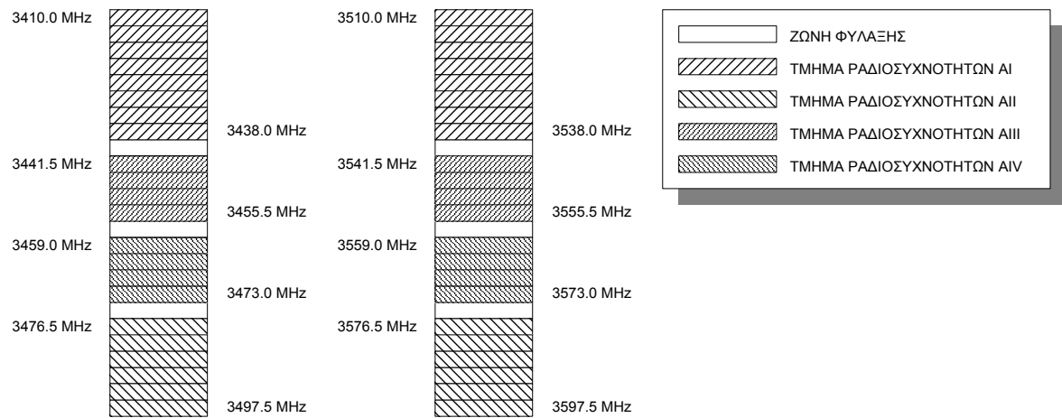
Σχήμα 2. Τμήματα Ραδιοσυχνοτήτων στη Φασματική Περιοχή των 25GHz
