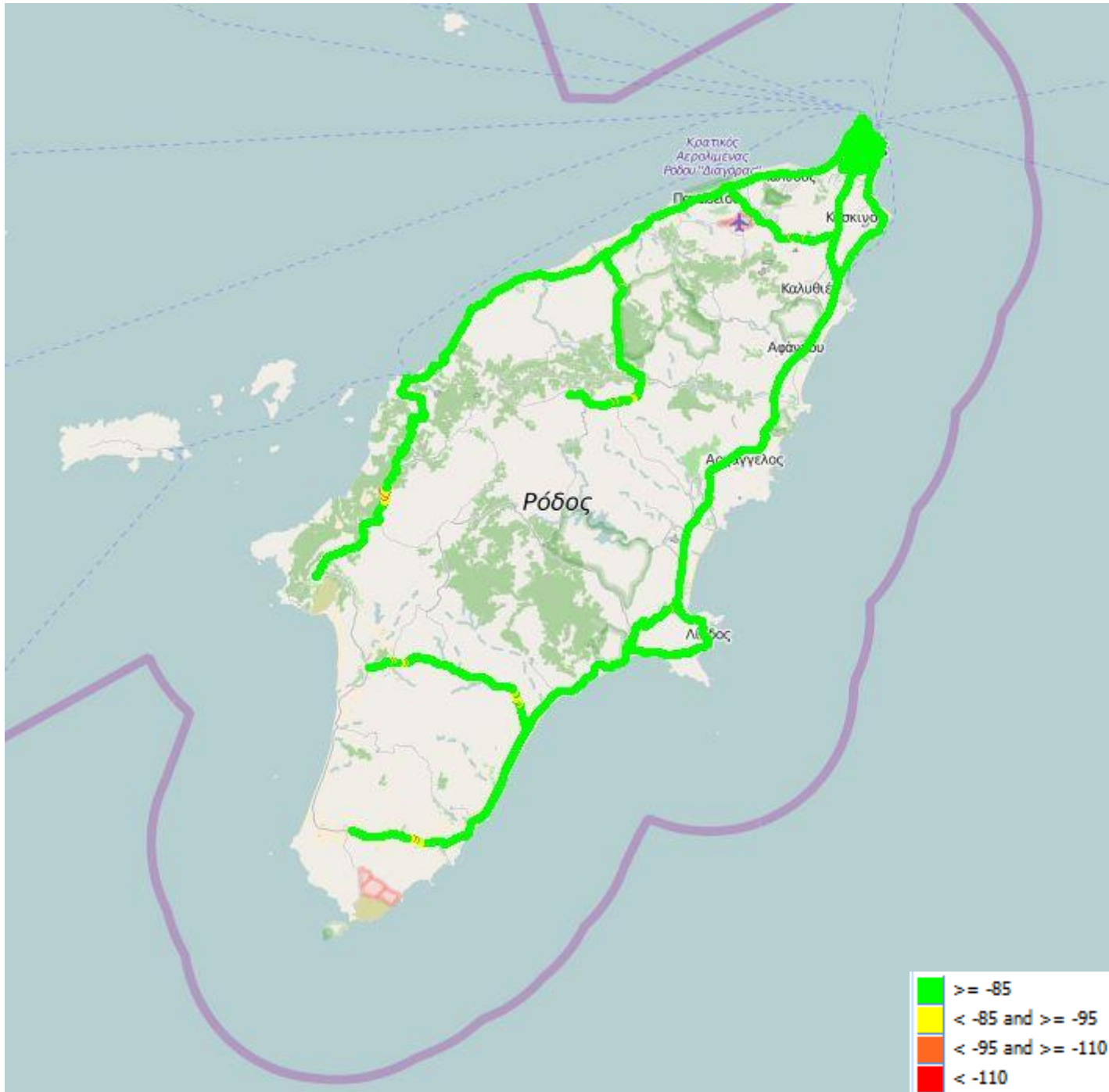
Εικόνα 13-3: Ραδιοκάλυψη WIND – GSM
