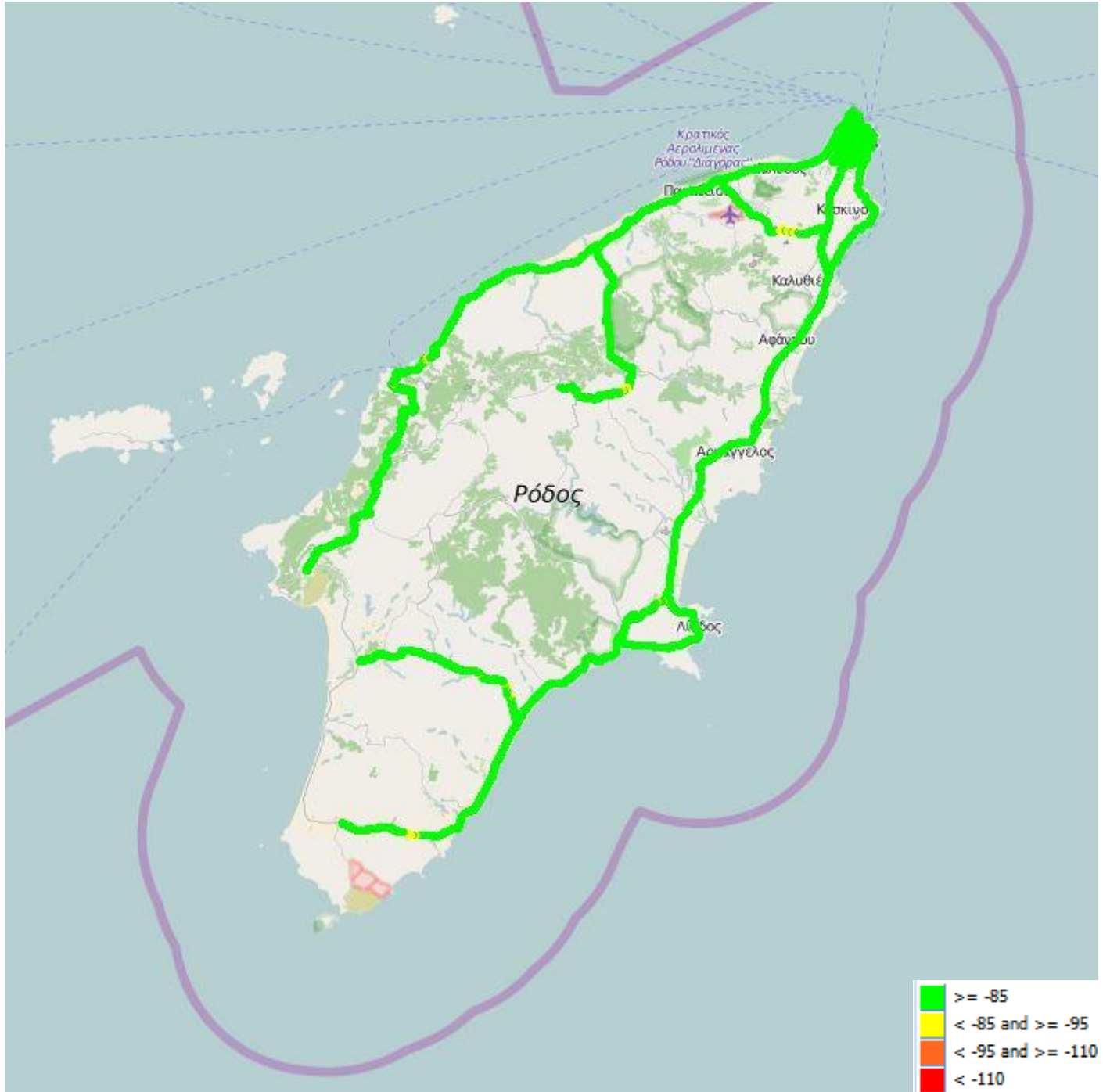
Εικόνα 13-1: Ραδιοκάλυψη Cosmote – GSM
