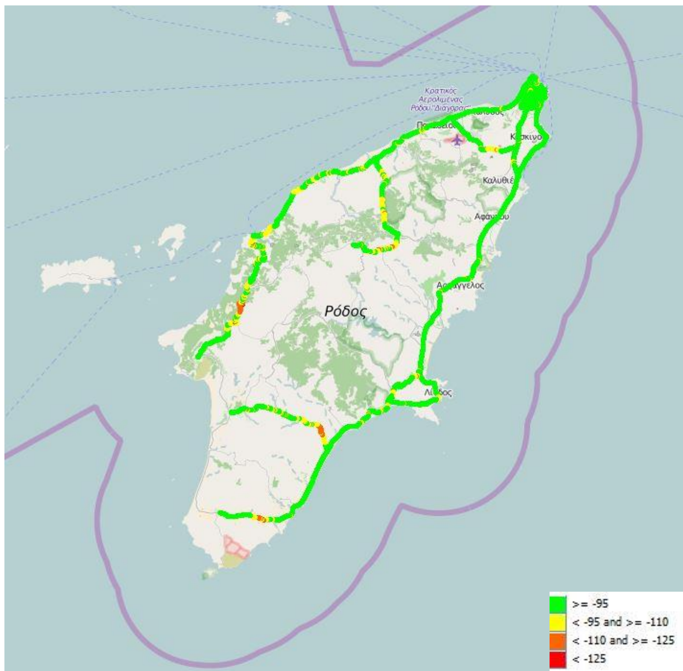
Εικόνα 13-9: Ραδιοκάλυψη Wind – LTE
