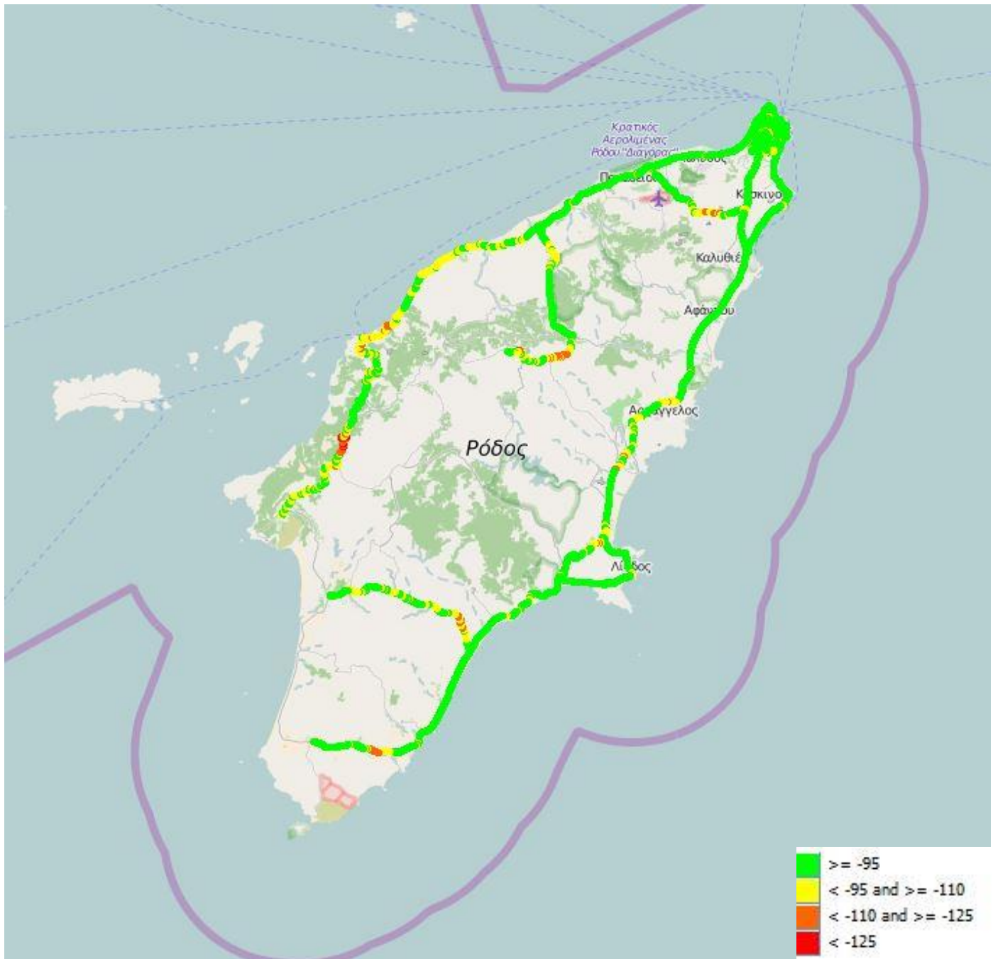
Εικόνα 13-7: Ραδιοκάλυψη Cosmote – LTE
