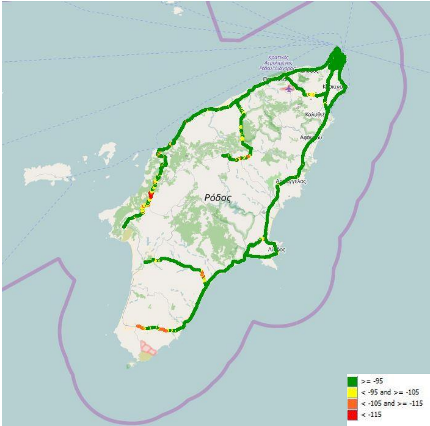
Εικόνα 13-5: Ραδιοκάλυψη Vodafone – UMTS
