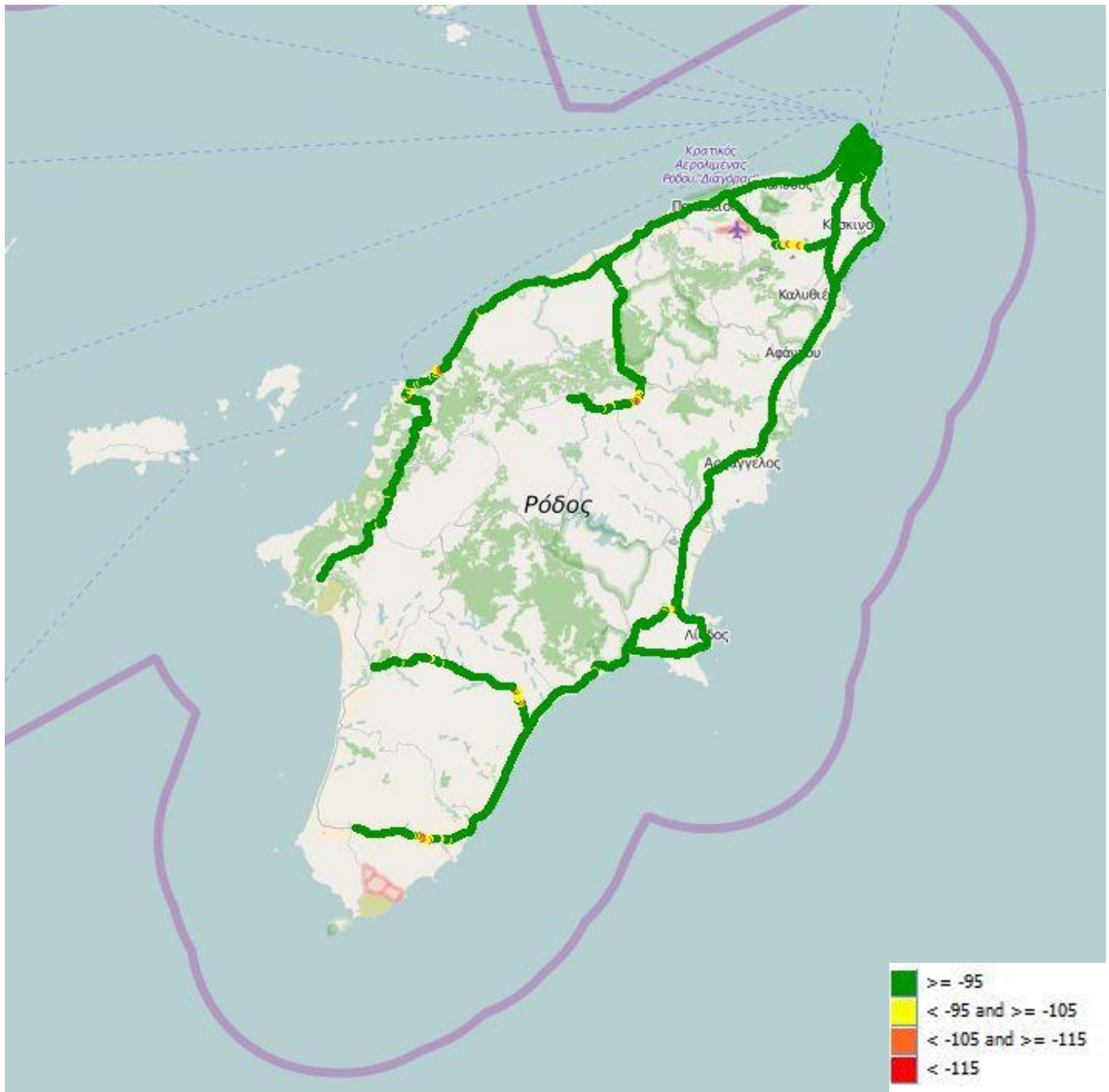
Εικόνα 13-4: Ραδιοκάλυψη Cosmote – UMTS
