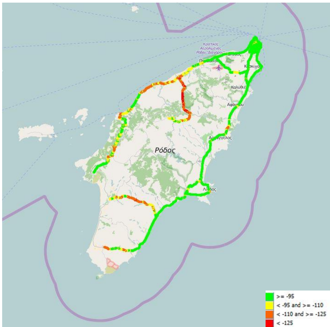
Εικόνα 13-8: Ραδιοκάλυψη Vodafone – LTE
