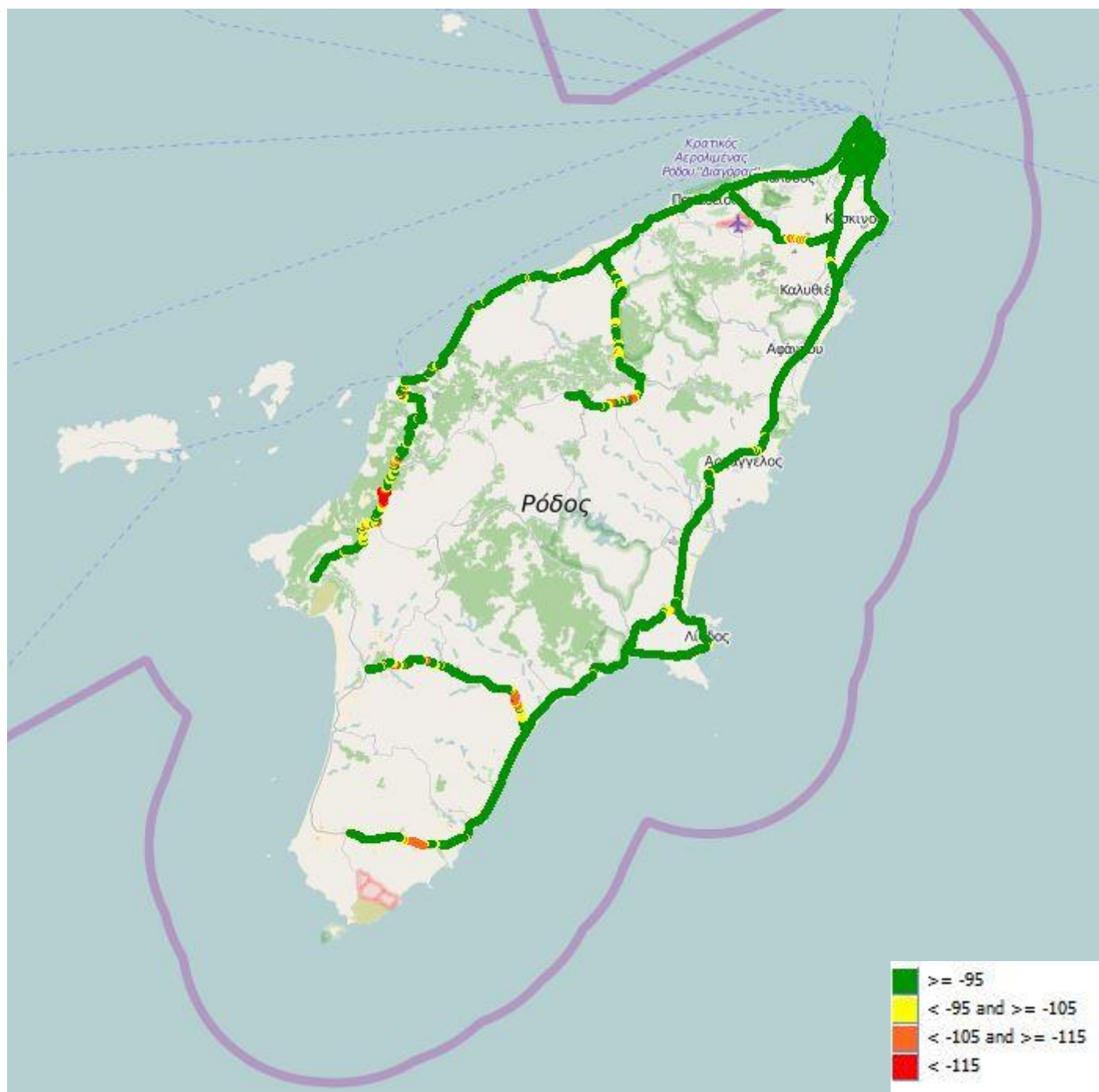
Εικόνα 13-6: Ραδιοκάλυψη WIND – UMTS
