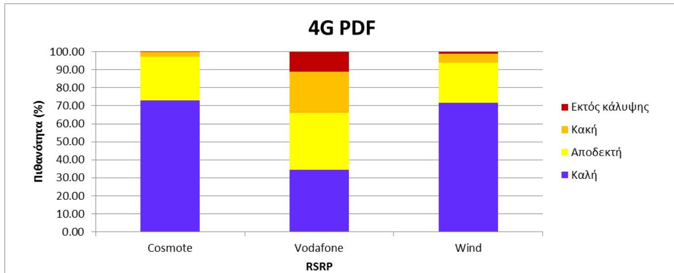
Εικόνα 14-3: Κατανομή Αθροιστικής Πυκνότητας Πιθανότητας Ραδιοκάλυψης LTE
