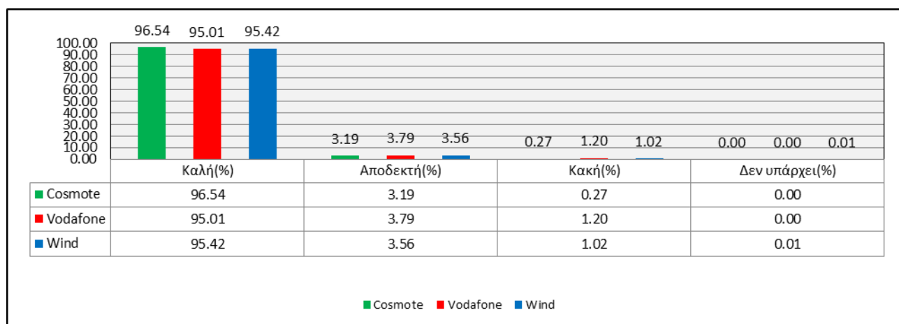
Εικόνα 3-2: Ποσοστό ραδιοκάλυψης (%)
