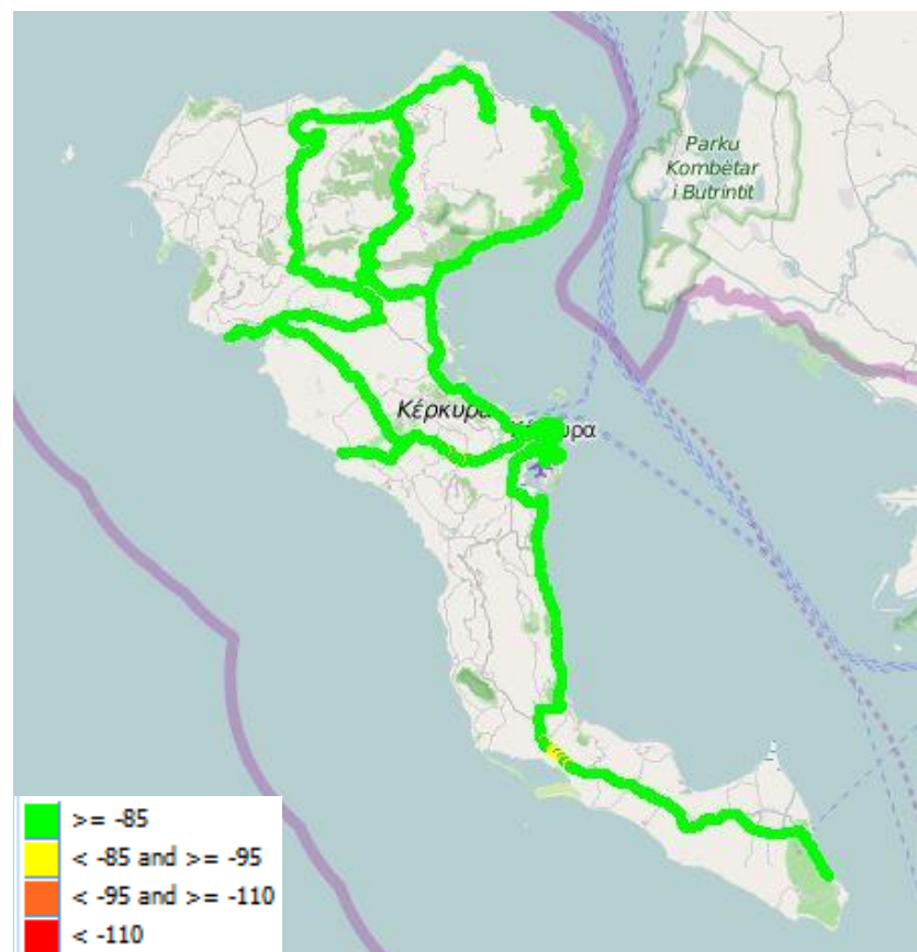
Εικόνα 13-1: Ραδιοκάλυψη Cosmote – GSM
