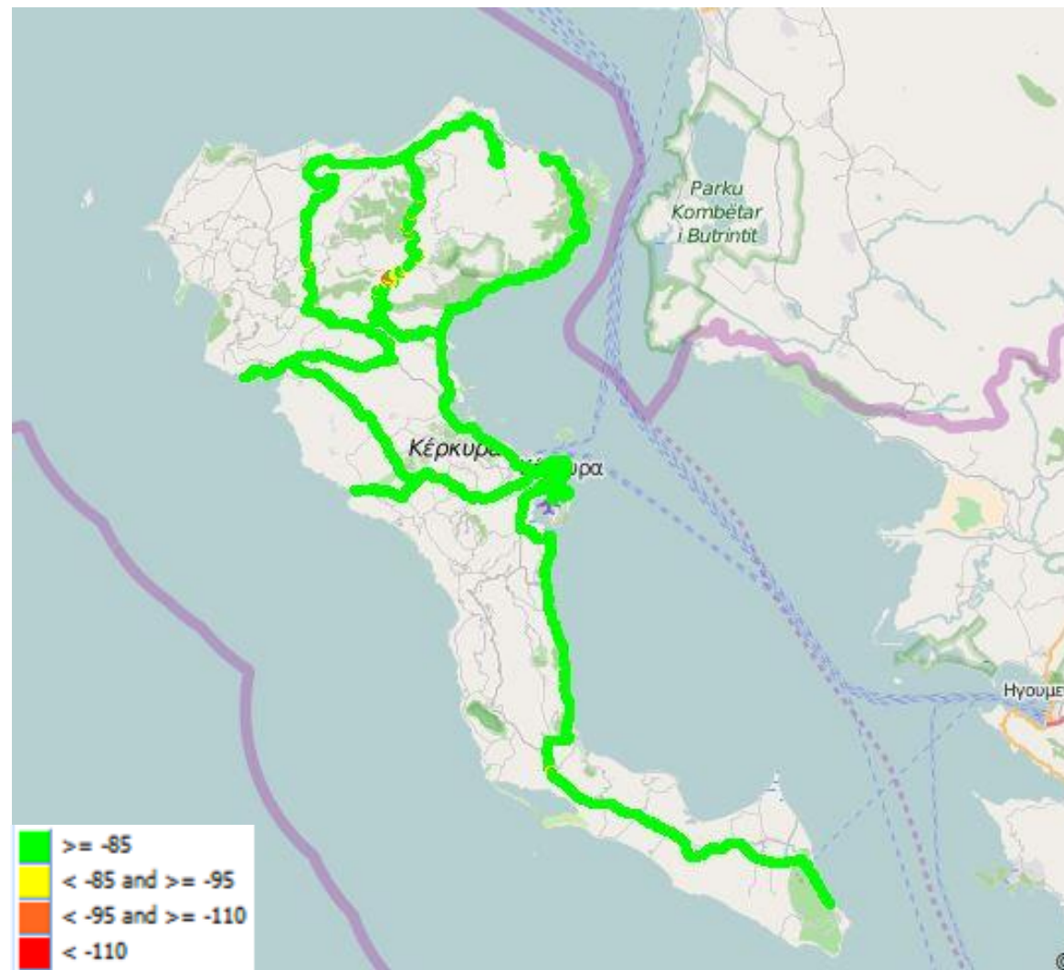
Εικόνα 13-2: Ραδιοκάλυψη Vodafone – GSM
