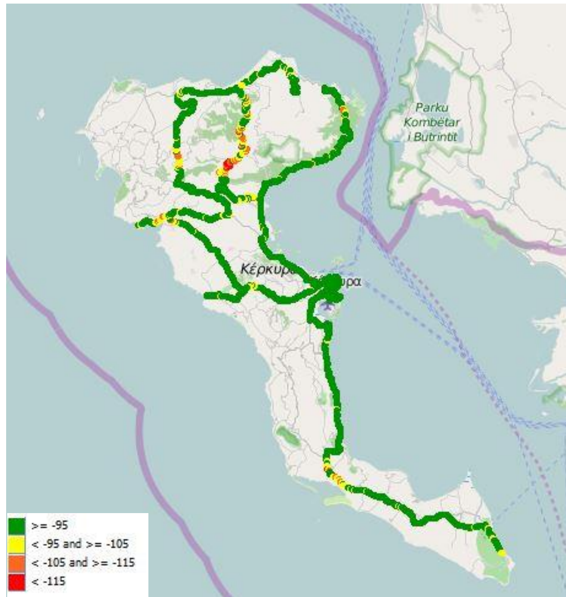
Εικόνα 13-5: Ραδιοκάλυψη Vodafone – UMTS
