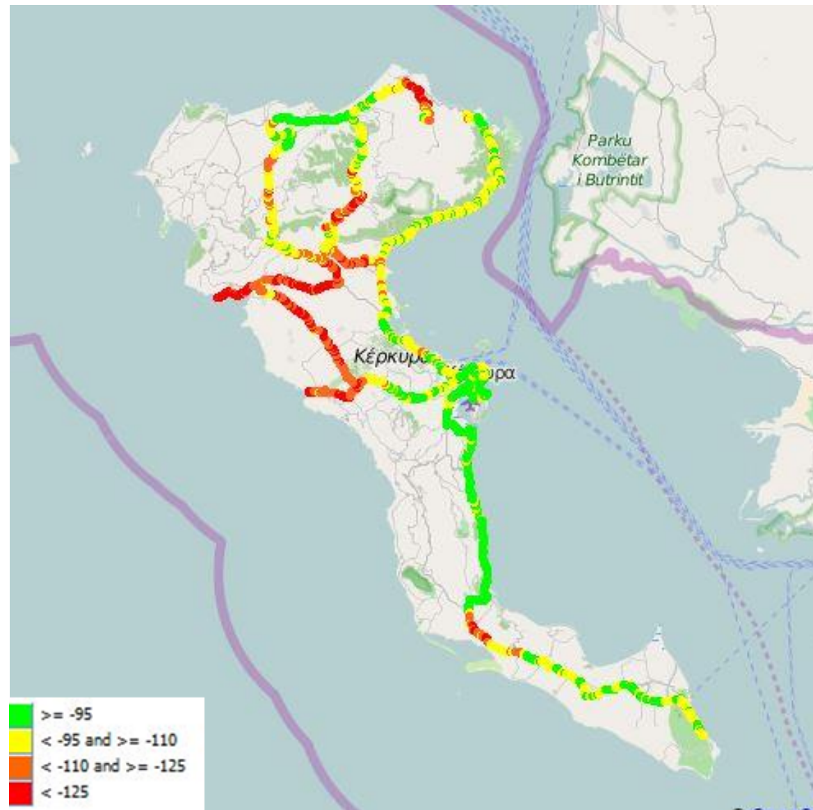
Εικόνα 13-8: Ραδιοκάλυψη Vodafone – LTE
