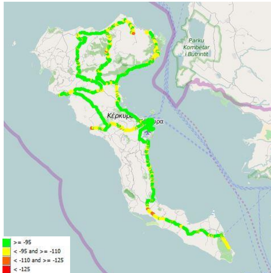
Εικόνα 13-7: Ραδιοκάλυψη Cosmote – LTE
