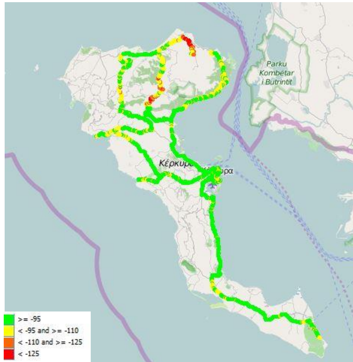
Εικόνα 13-9: Ραδιοκάλυψη Wind – LTE
