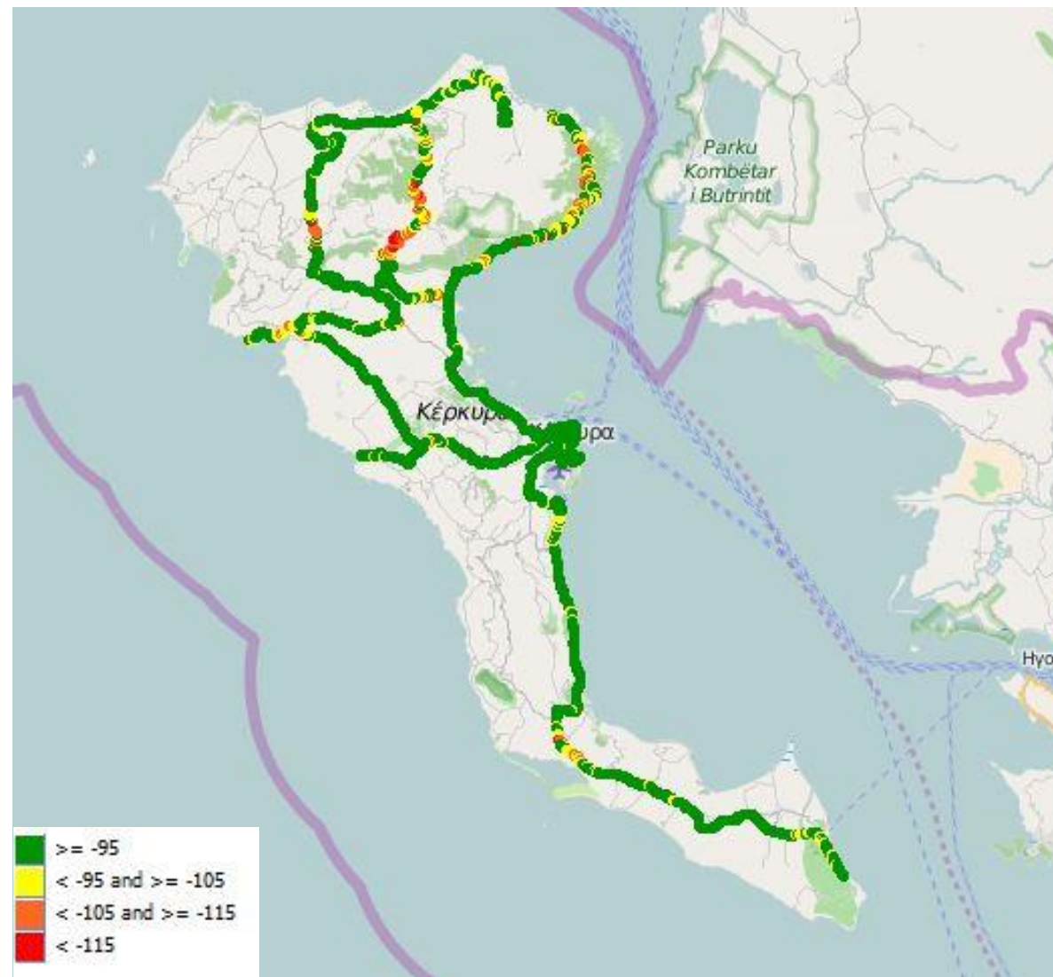
Εικόνα 13-6: Ραδιοκάλυψη WIND – UMTS
