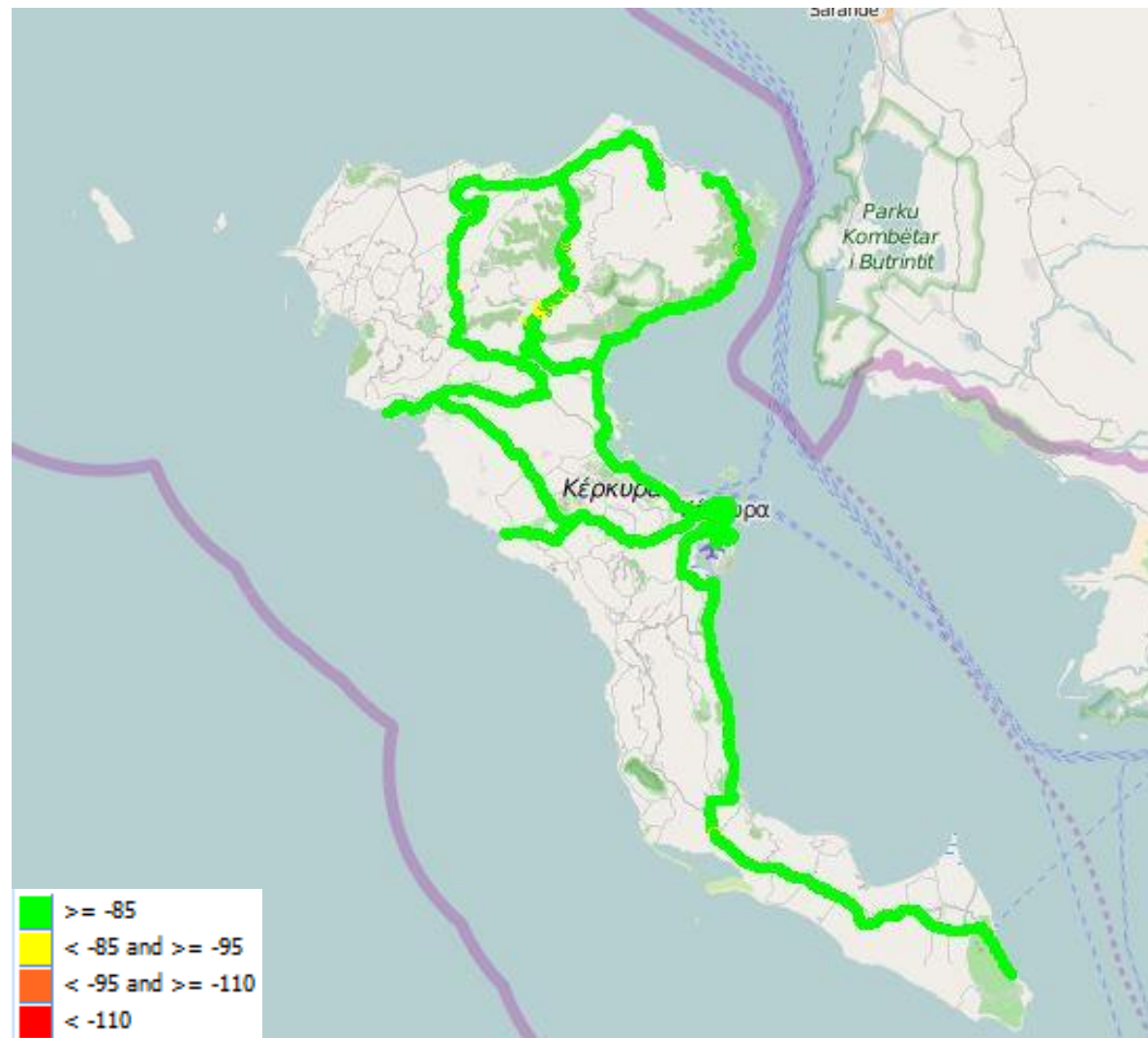
Εικόνα 13-3: Ραδιοκάλυψη WIND – GSM
