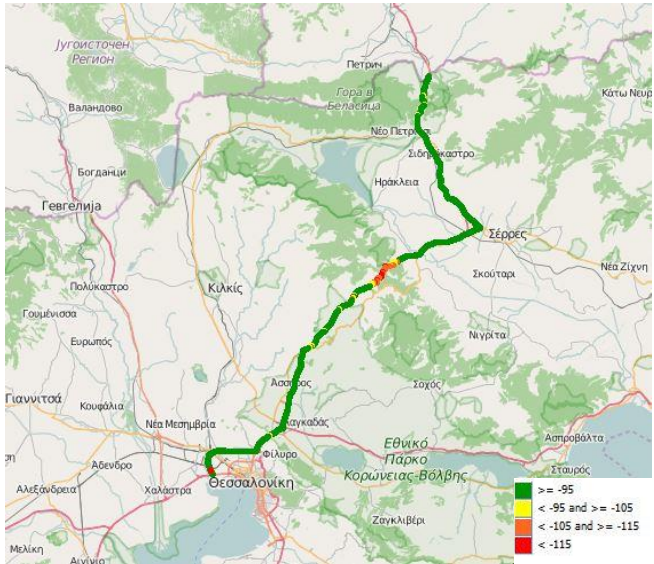
Εικόνα 13-5: Ραδιοκάλυψη Vodafone – UMTS
