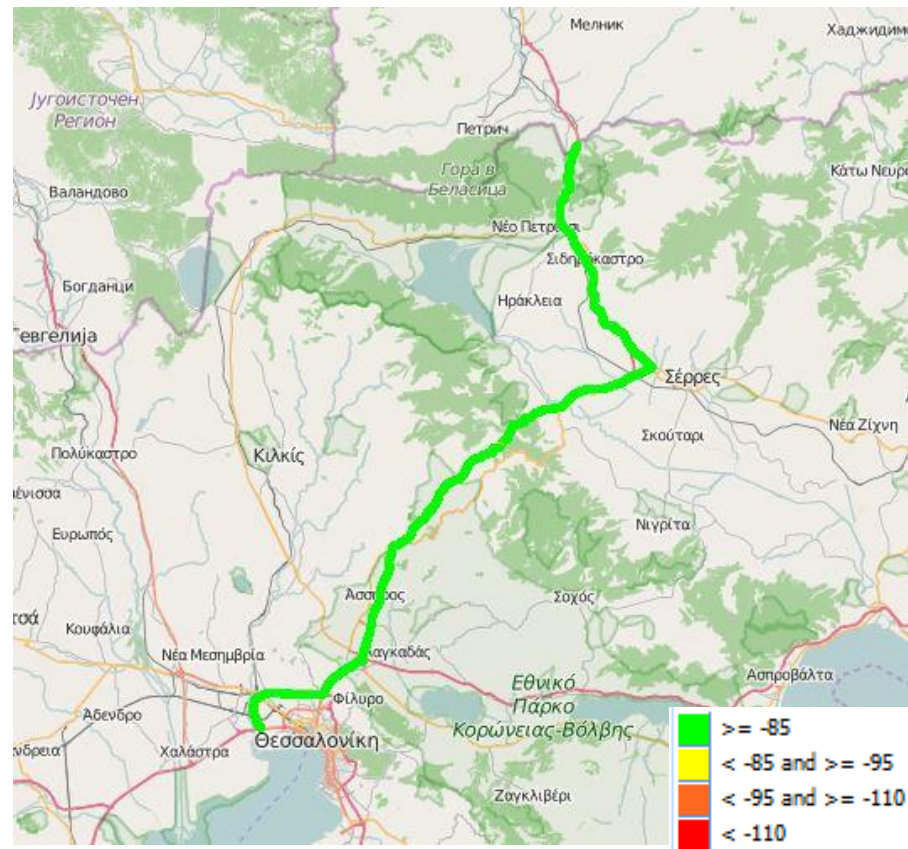
Εικόνα 13-1: Ραδιοκάλυψη Cosmote – GSM
