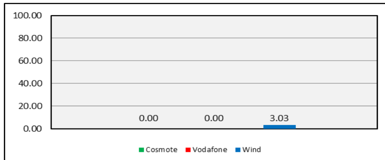
Εικόνα 5-5: Πιθανότητα διακοπής κλήσης φωνής (%)
