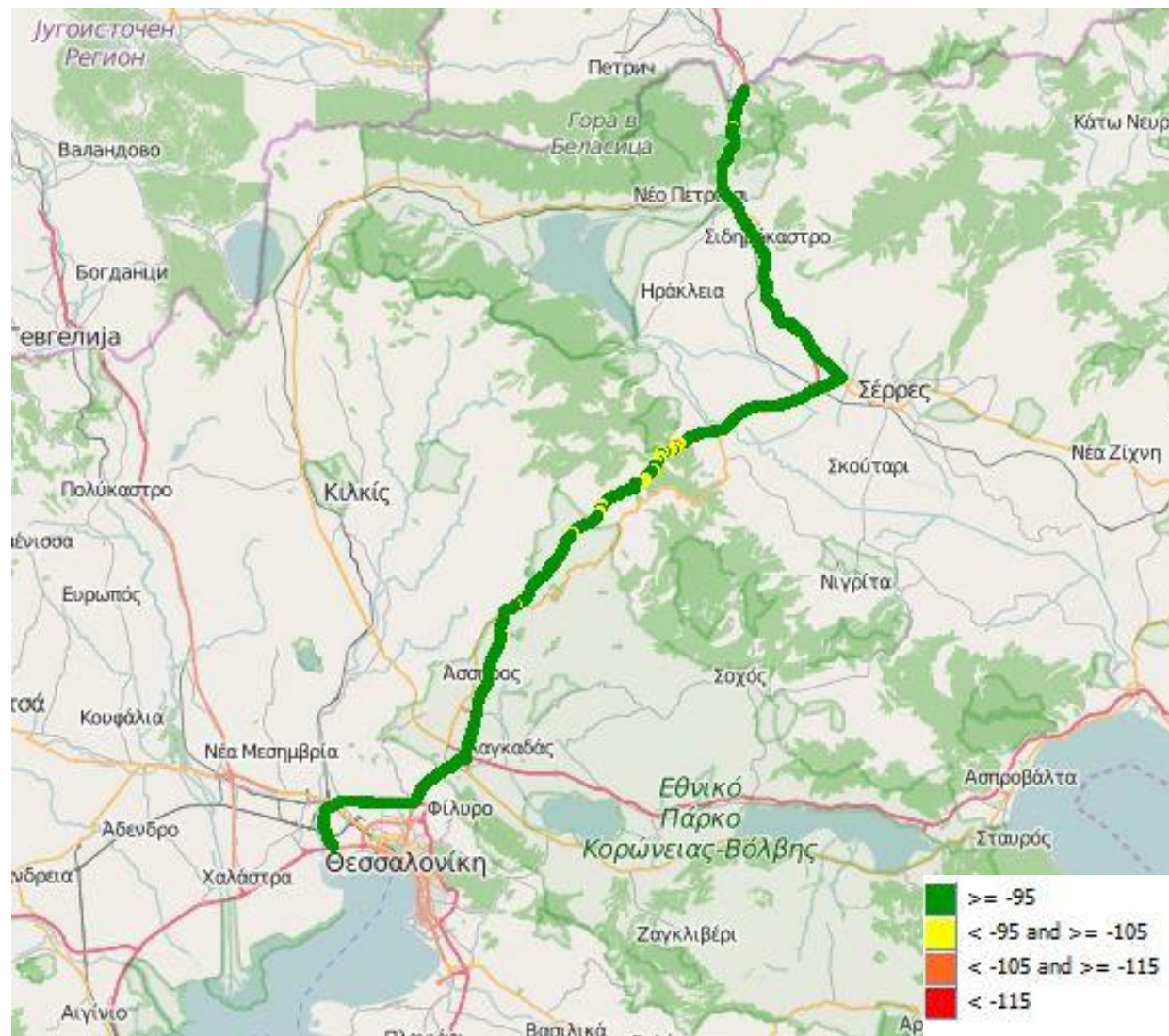
Εικόνα 13-4: Ραδιοκάλυψη Cosmote – UMTS
