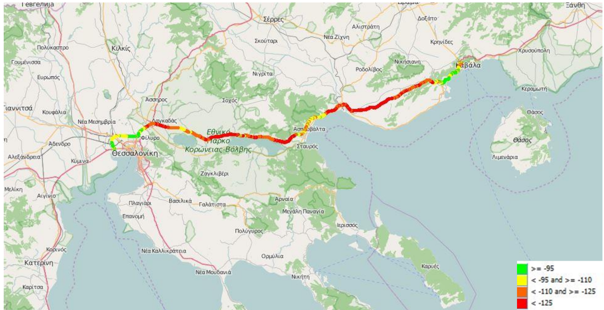
Εικόνα 13-8: Ραδιοκάλυψη Vodafone – LTE
