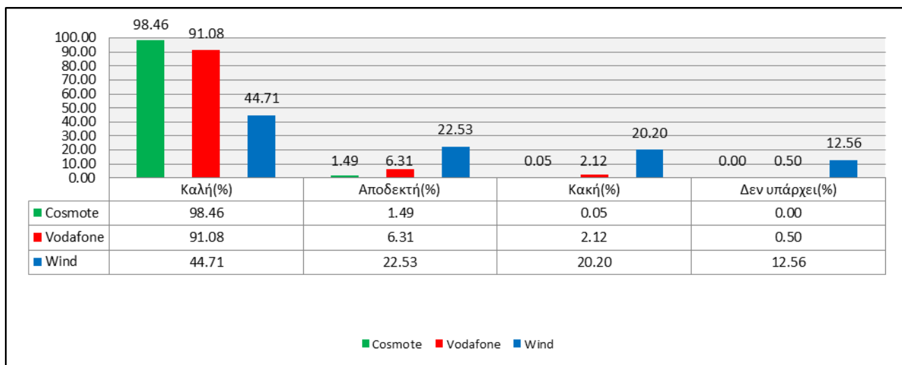
Εικόνα 3-4: Ποσοστό ραδιοκάλυψης (%)
