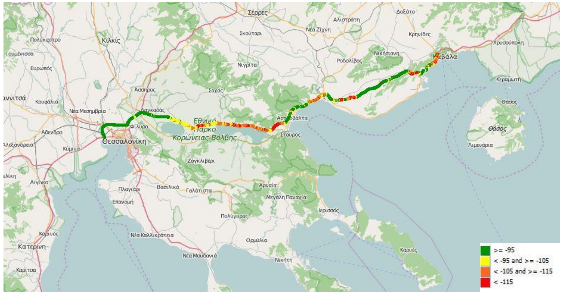
Εικόνα 13-6: Ραδιοκάλυψη WIND – UMTS
