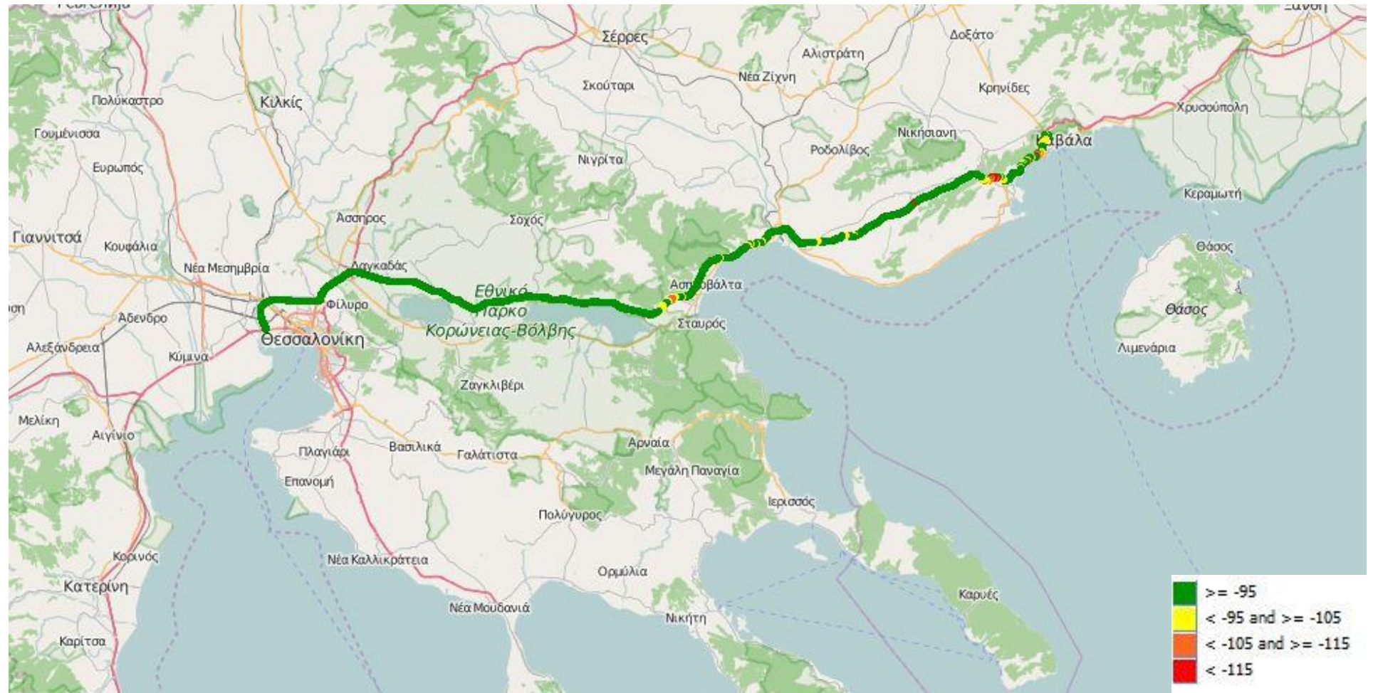
Εικόνα 13-5: Ραδιοκάλυψη Vodafone – UMTS
