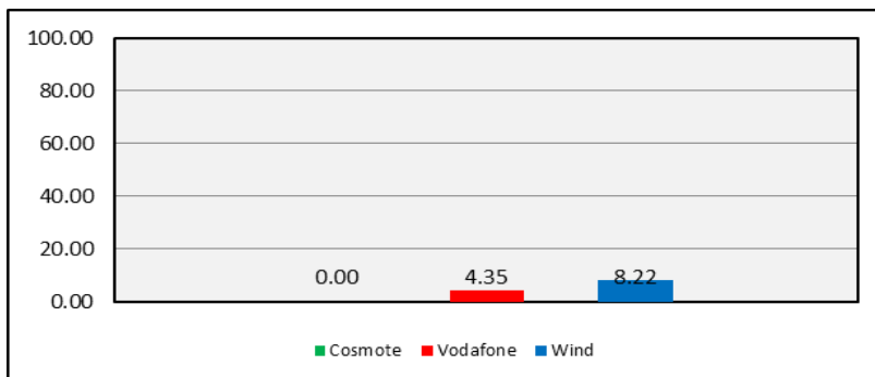
Εικόνα 5-5: Πιθανότητα διακοπής κλήσης φωνής (%)
