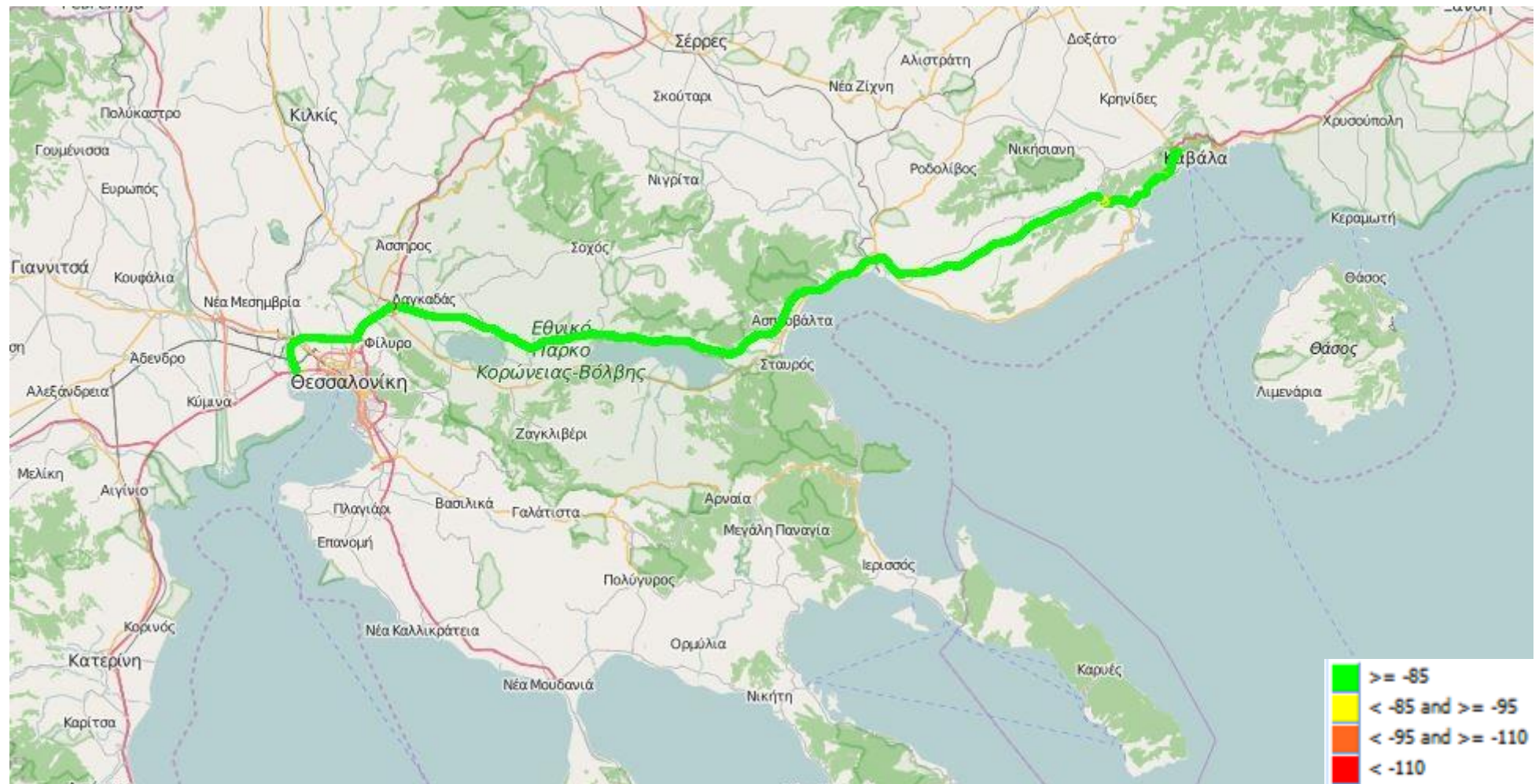
Εικόνα 13-2: Ραδιοκάλυψη Vodafone – GSM
