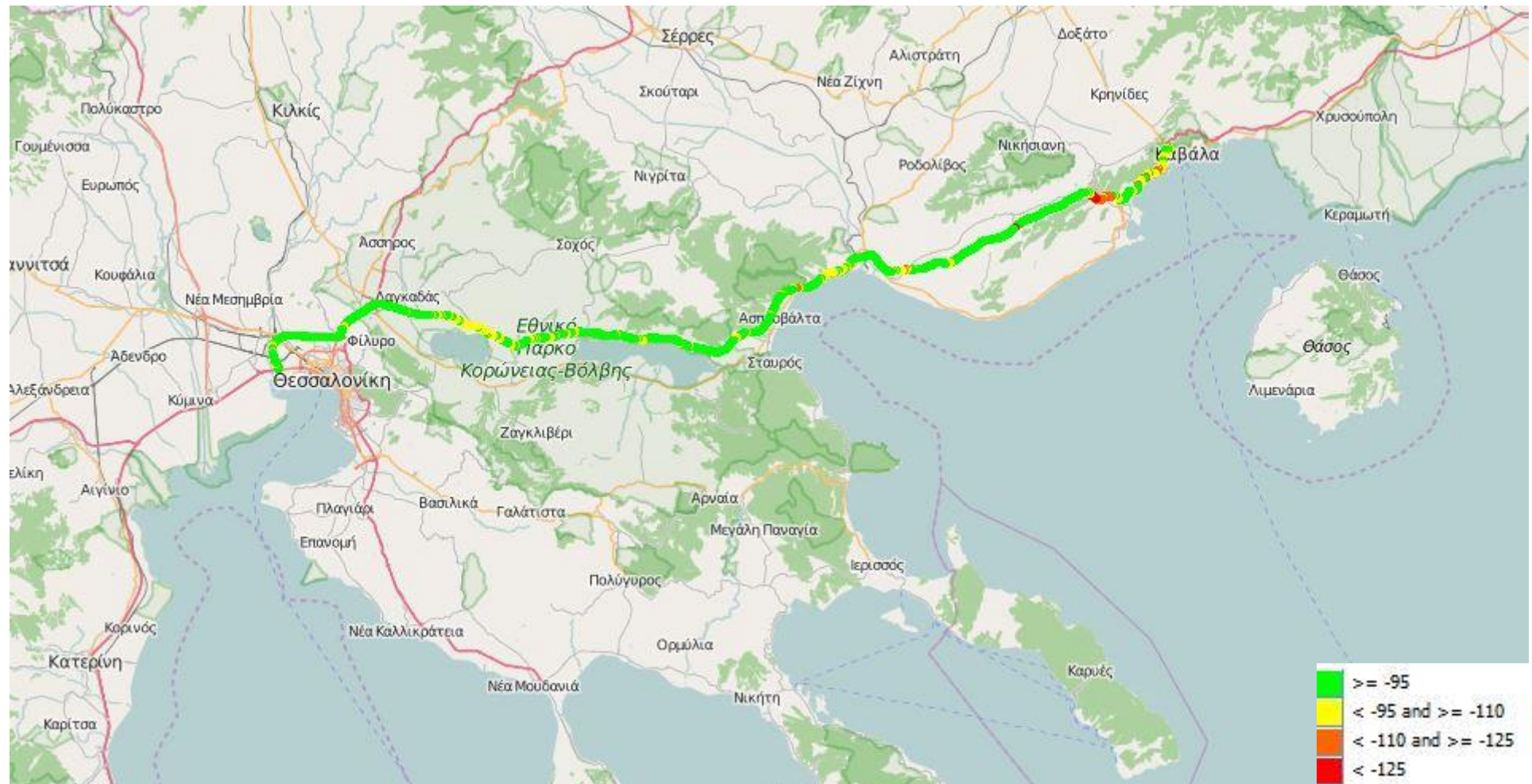
Εικόνα 13-7: Ραδιοκάλυψη Cosmote – LTE
