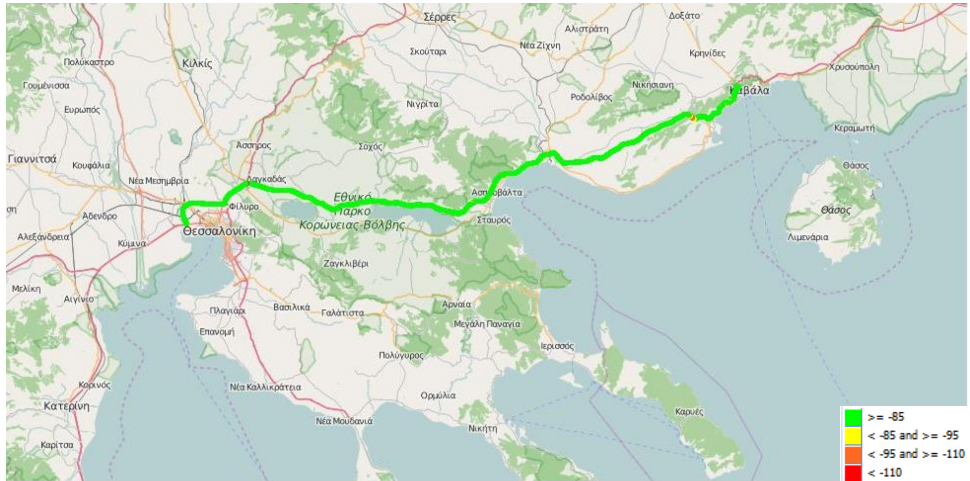
Εικόνα 13-3: Ραδιοκάλυψη WIND – GSM
