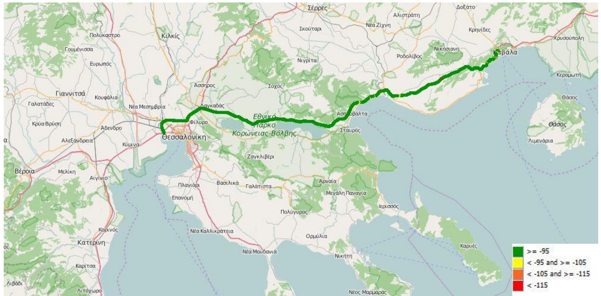
Εικόνα 13-4: Ραδιοκάλυψη Cosmote – UMTS
