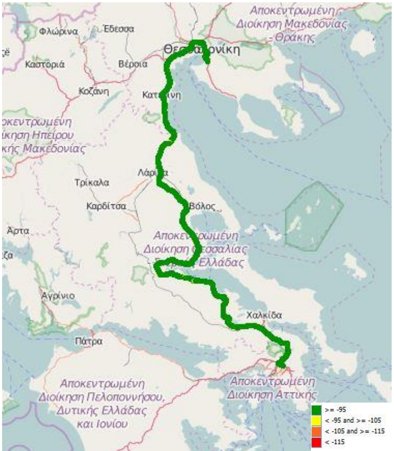
Εικόνα 13-4: Ραδιοκάλυψη Cosmote – UMTS
