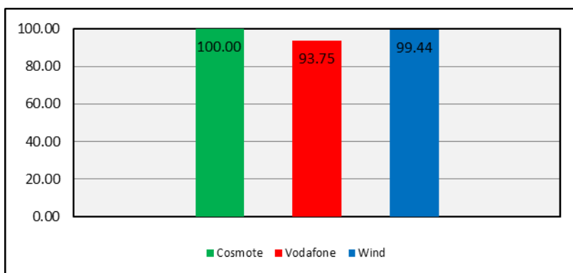
Εικόνα 5-4: Πιθανότητα διατήρησης της κλήσης (%)
