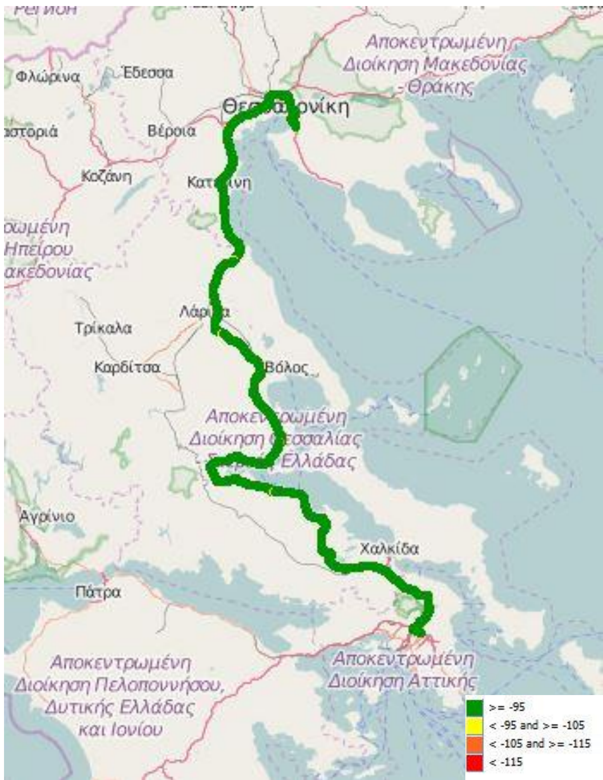
Εικόνα 13-5: Ραδιοκάλυψη Vodafone – UMTS
