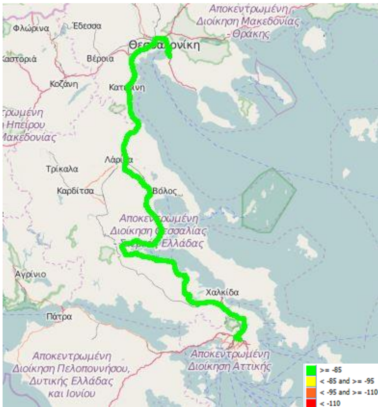
Εικόνα 13-2: Ραδιοκάλυψη Vodafone – GSM
