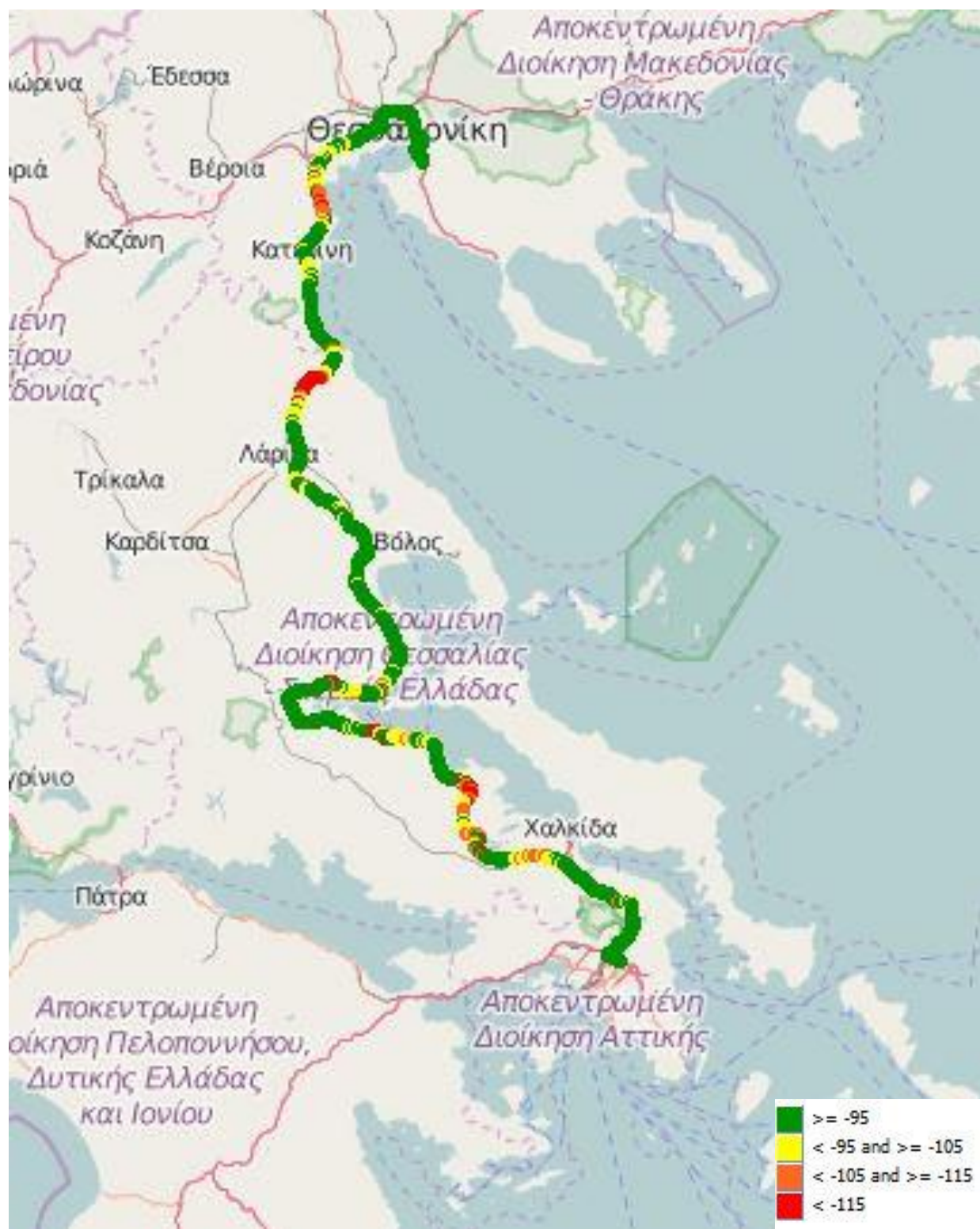
Εικόνα 13-6: Ραδιοκάλυψη WIND – UMTS
