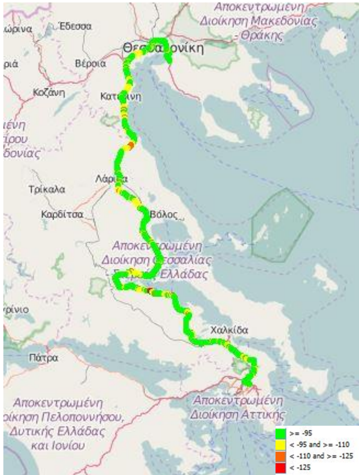
Εικόνα 13-7: Ραδιοκάλυψη Cosmote – LTE
