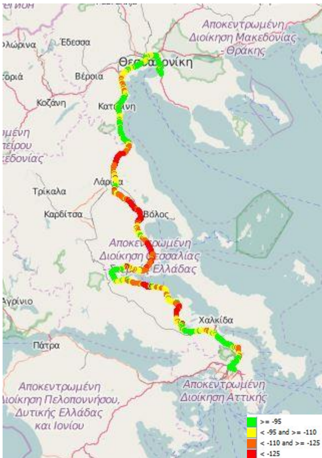
Εικόνα 13-8: Ραδιοκάλυψη Vodafone – LTE
