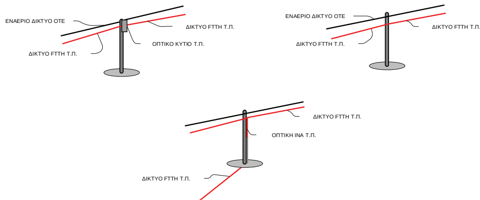
Σχήμα 6. Ενδεικτική απεικόνιση της υπηρεσίας πρόσβασης σε στύλους ΟΤΕ.
