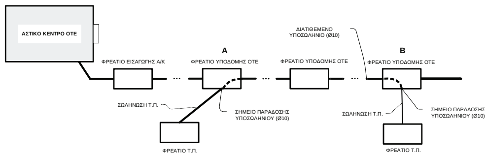
Σχήμα 1. Διάγραμμα παροχής σωληνώσεων ΟΤΕ σε Τ.Π. Ο Τ.Π. παραλαμβάνει υποσωληνία από τα σημεία Α & Β (Φρεάτια υποδομής ΟΤΕ που βρίσκονται πλησιέστερα στα σημεία επιλογής του Τ.Π.). Τα φρεάτια αλλά και η παρεχόμενη σωλήνωση βρίσκονται εντός διαδρομής όπως αυτή απεικονίζεται στη βάση ΧΕΜΔ.
